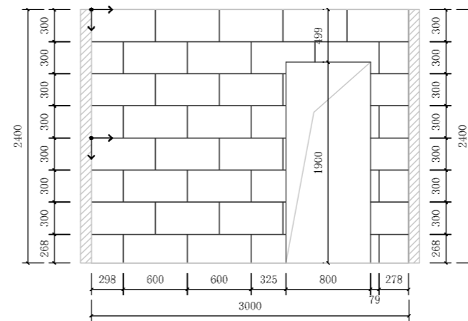
D Bathroom D Front Ele 1:50
