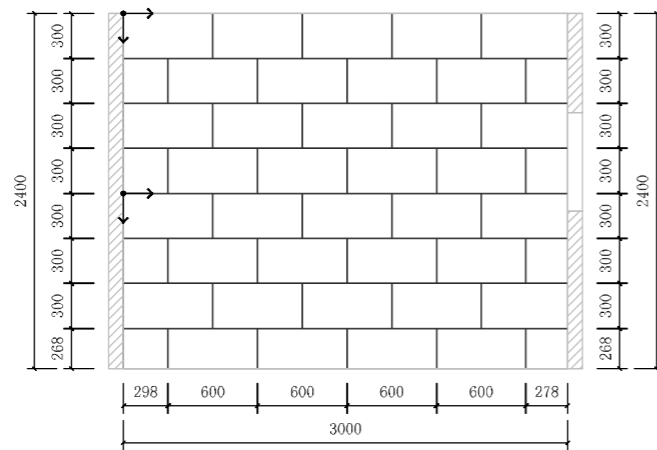
B Bathroom B Front Ele 1:50
