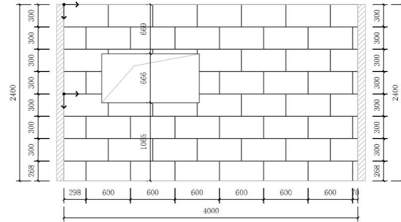
C Bathroom C Front Ele 1:50
